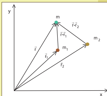
Figura 3.5. Coordenadas de posición de m_1 y m_2 donde r_i = |\vec{r} - \vec{r}_i| .
