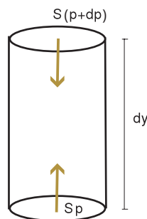
Figura 3.4. Cilindro de base S y altura dy .
